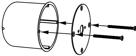
1C Montage über Unterputzdose Installation via flush-mounted box
